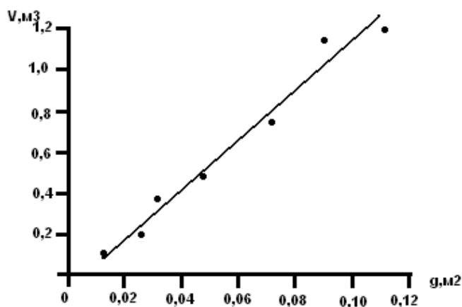
Рис.3 Прямая объемов
