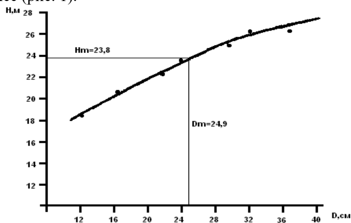
Рис.1 Кривая высот
